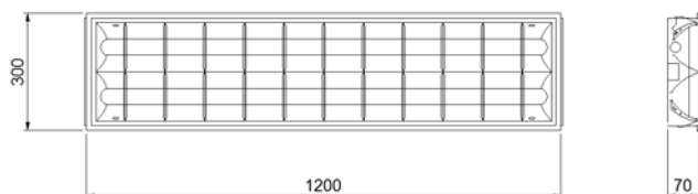
KIT-S OFFISIMPLE T8 236 W
