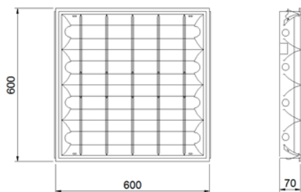
KIT-S OFFISIMPLE T8 418 W
